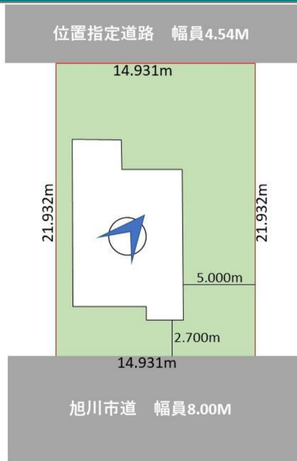
地籍図
